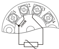
Rys. 3.3 Podłączenie czujnika Pt100, Ni100 2-przewodowe
