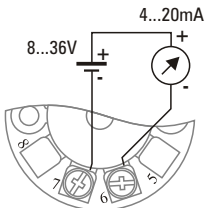
Rys. 3.5 Podłączenie wyjścia 4...20 mA (TEH-27, TEH-28)
