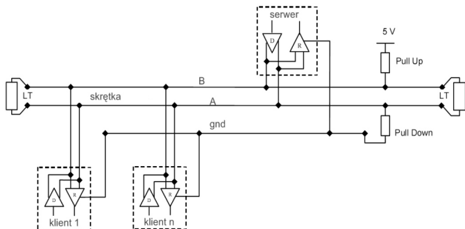
Rys. 2.5 Zalecany sposób podłączenia interfejsu RS-485 Modbus-RTU
