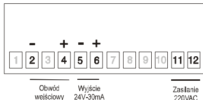
Listwa zaciskowa miernika
